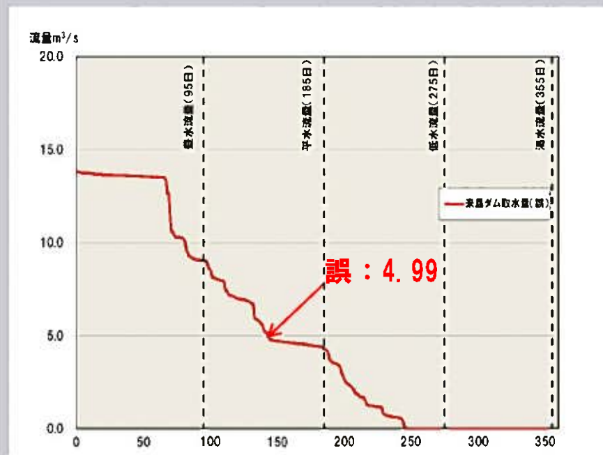
図-1 平成24年 来島ダム取水量流況 (誤)
