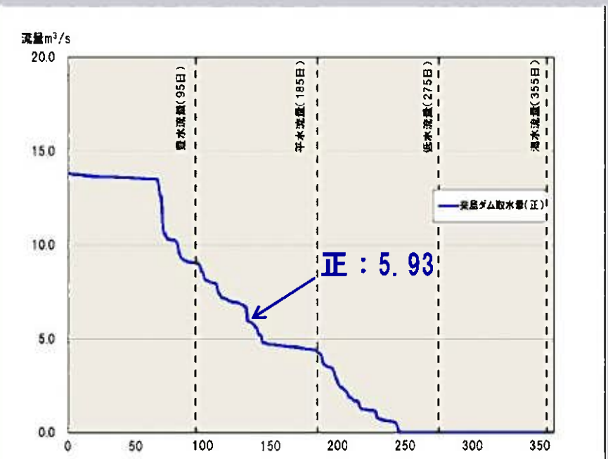
図-2 平成24年 来島ダム取水量流況 (正)
