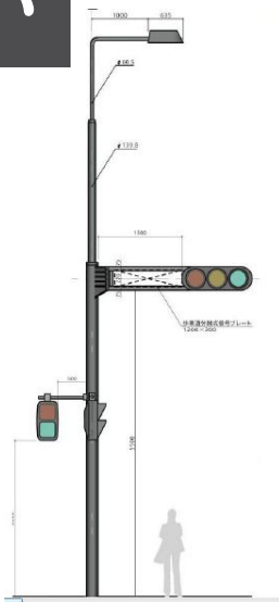
信号機
