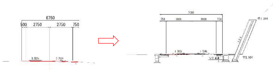
標準断面図
