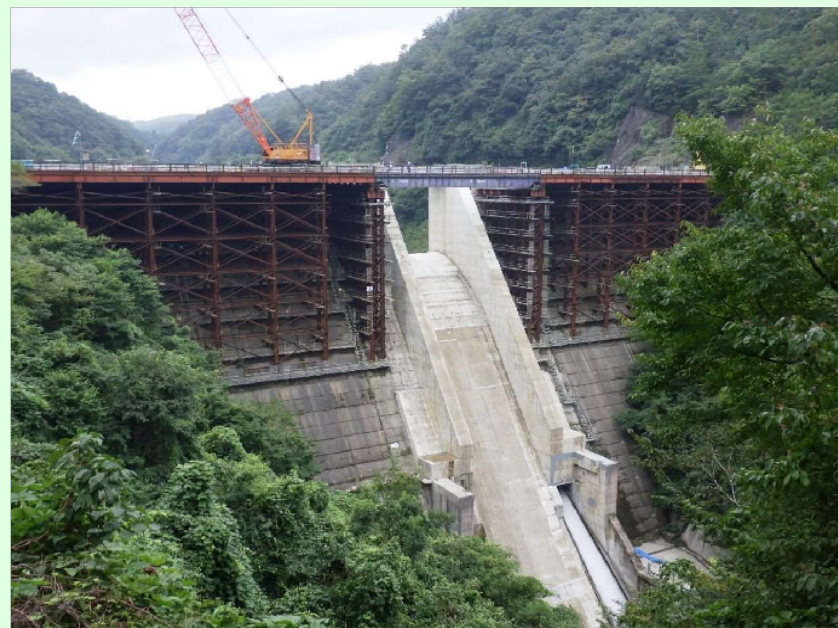
堤体下流面
