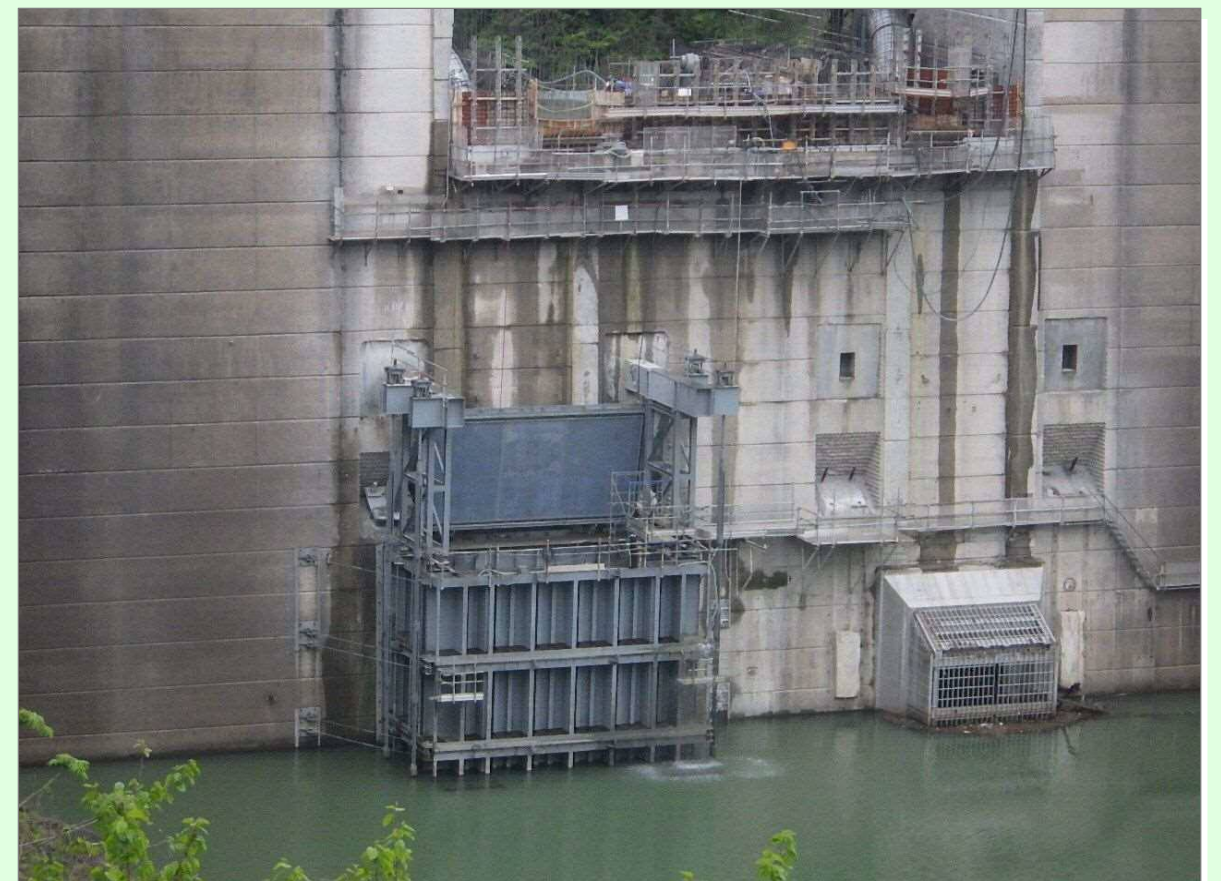
左岸仮締切
