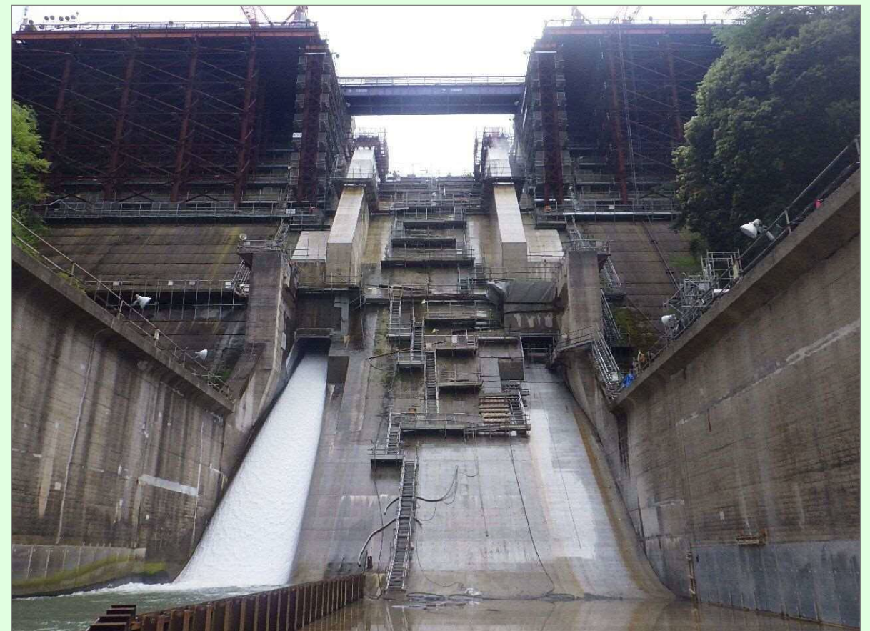
堤体下流面2
