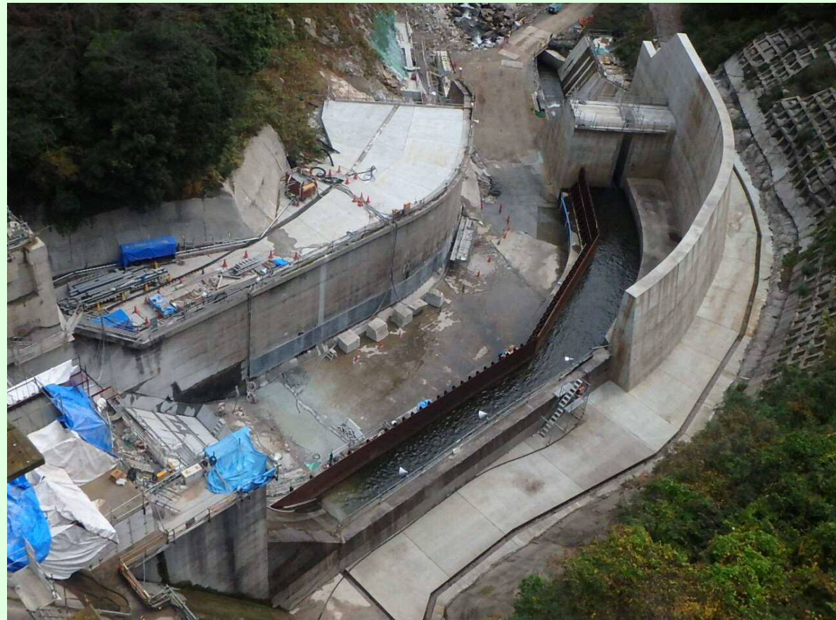
減勢工1
