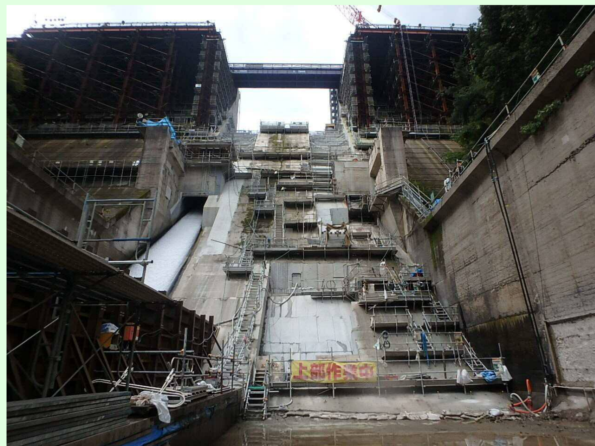
堤体下流面2
