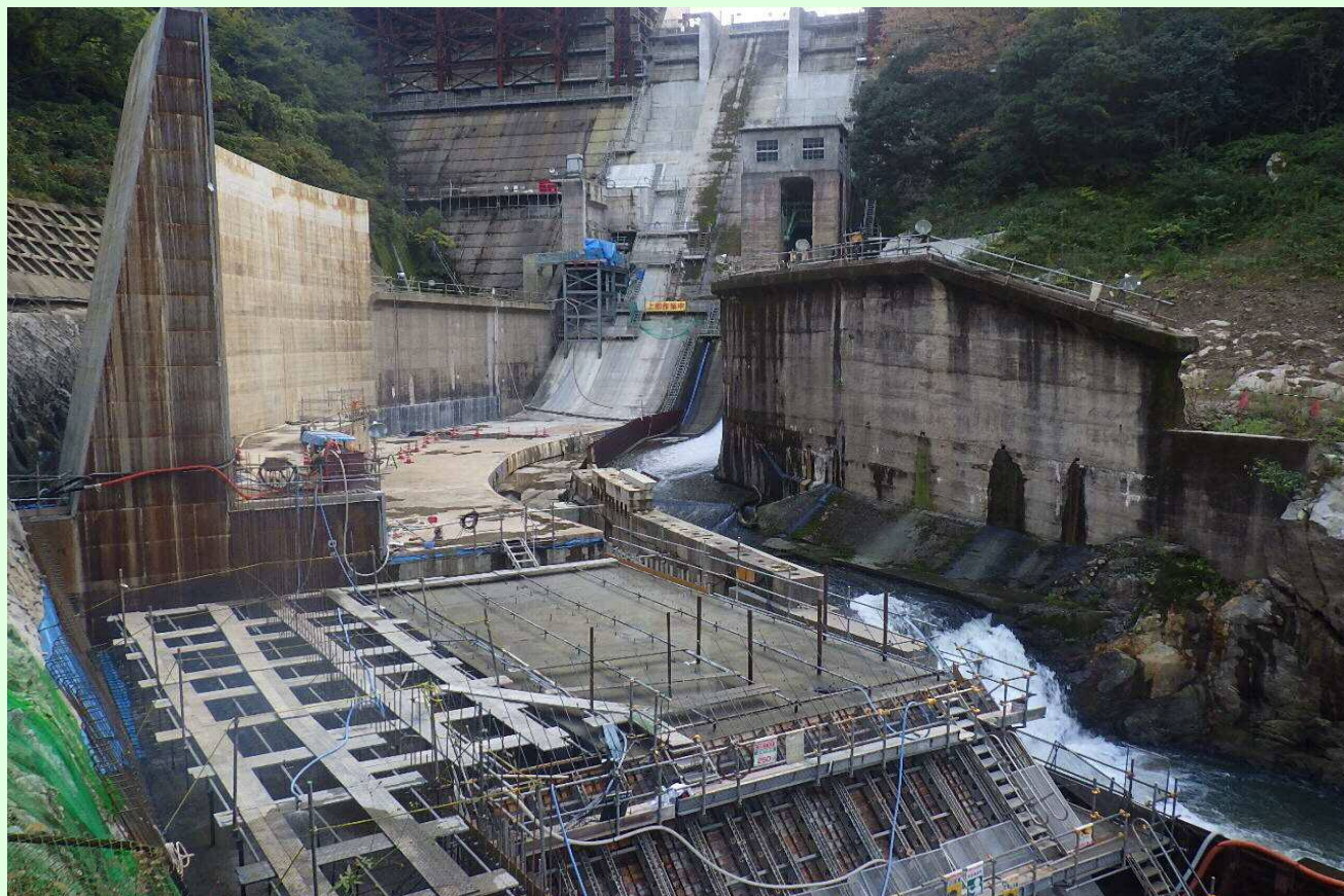
右岸副ダム施工状況
