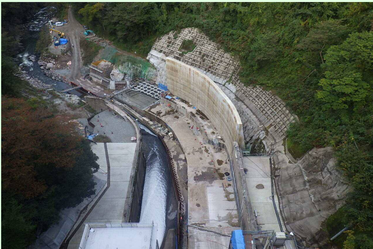
減勢工・工事用道路
