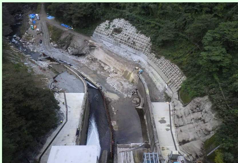
減勢工・工事用道路
