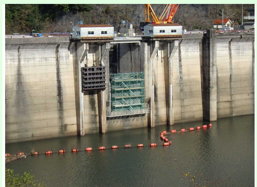
堤頂部既設取壊し状況
