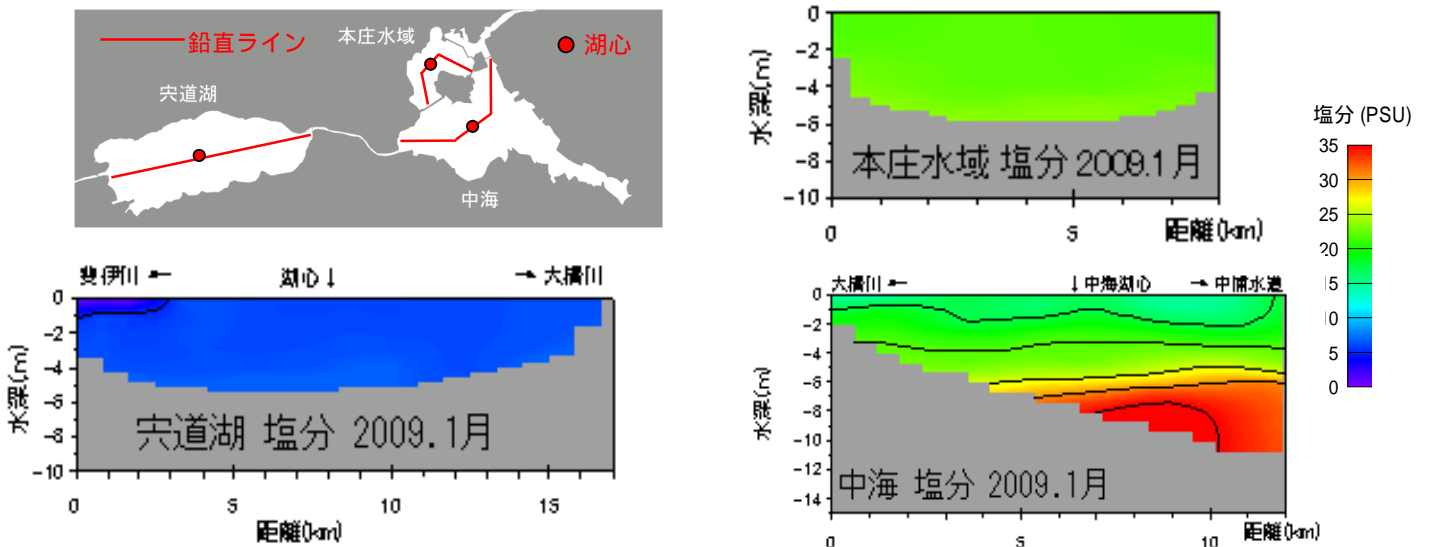
塩分 鉛直分布
