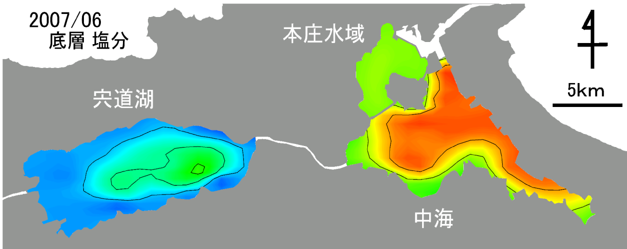
底層塩分 水平分布
