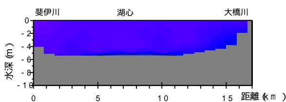
宍道湖 塩分 2003.10月
