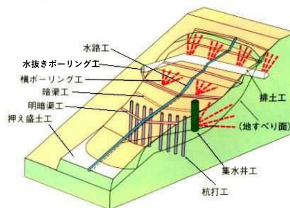
■対策工法の模式図
