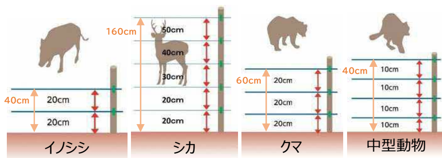
〈電気柵の標準図〉
