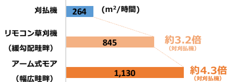
【アーム式モアによる機械除草】
