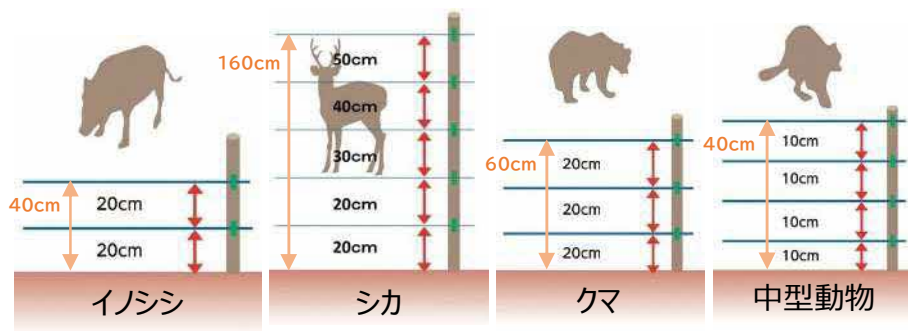
〈電気柵の標準図〉
