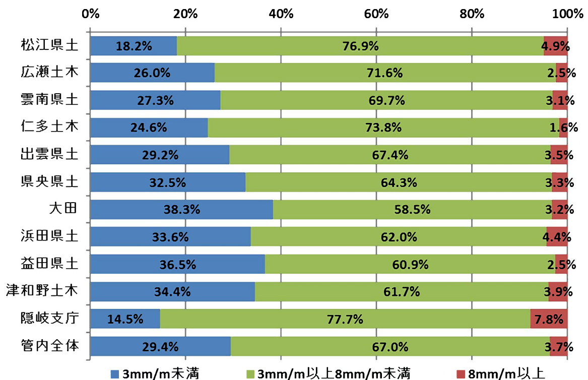
図 2-2-2 島根県管理道路の路面状況（IRI）
