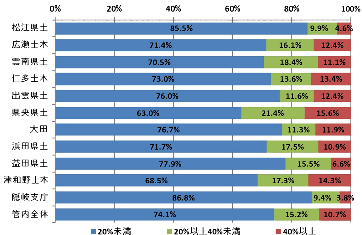
図 2-2-1 島根県管理道路の路面状況（ひび割れ率）
