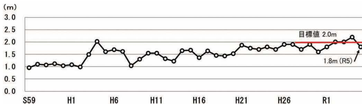
図1-6 米子湾の透明度の経年変化
