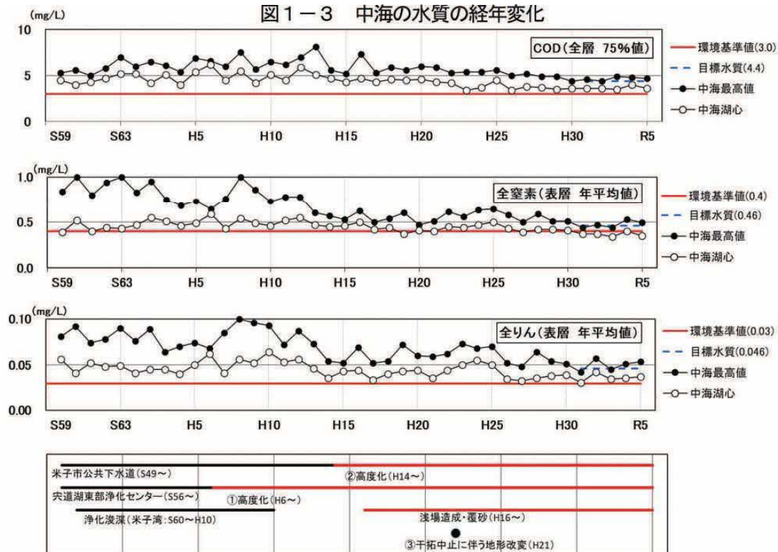
図1-3 中海の水質の経年変化
