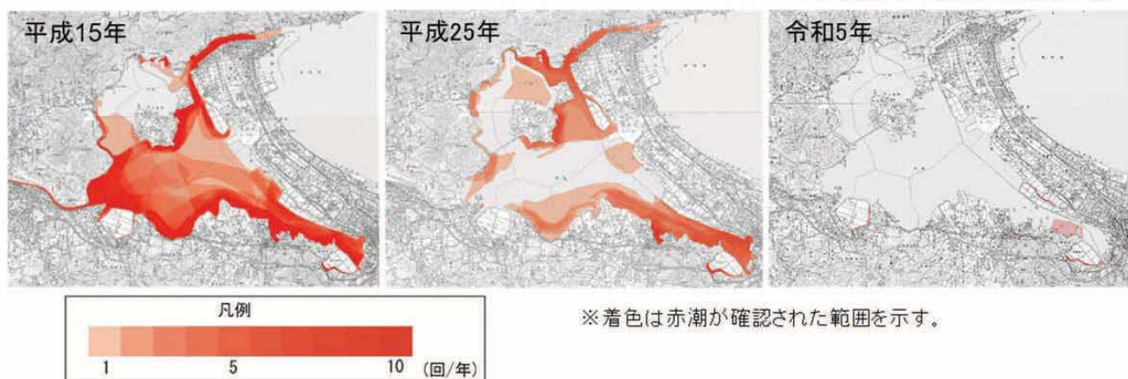
図1-4 中海の赤潮発生の回数と範囲
