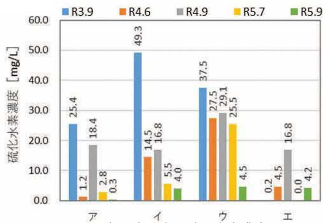
図4 各調査地点の硫化水素濃度
