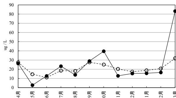
図2-2 宍道湖のクロロフィルa(Chl-a)の月別変化
