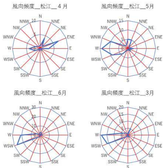
図 3 2023 年度の松江の光化学 0x 濃度 0.06ppm 以上観測時における風向頻度
