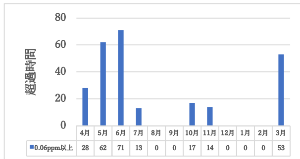
図 1 2023年度の松江において光化学 O_x の1時間値が 0.06\text{ppm} を超過した時間数
