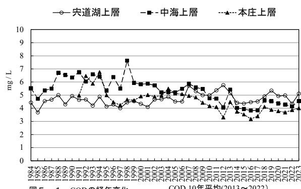
図 5-1 CODの経年変化
