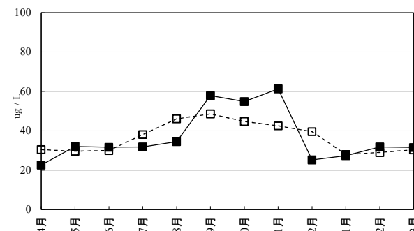
図3-4 中海の全リン(T-P)の月別変化
