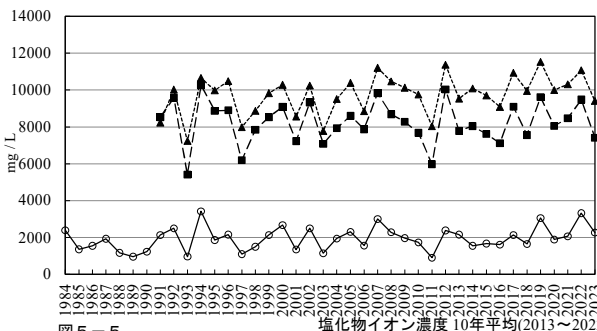
図 5-5 塩化物イオン濃度の経年変化
