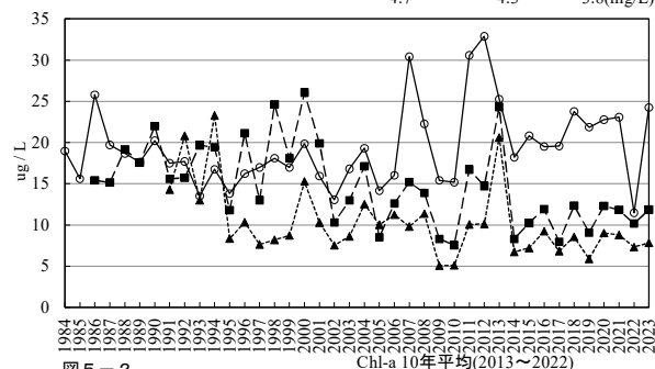
図 5-2 クロロフィルa(Chl-a)の経年変化
