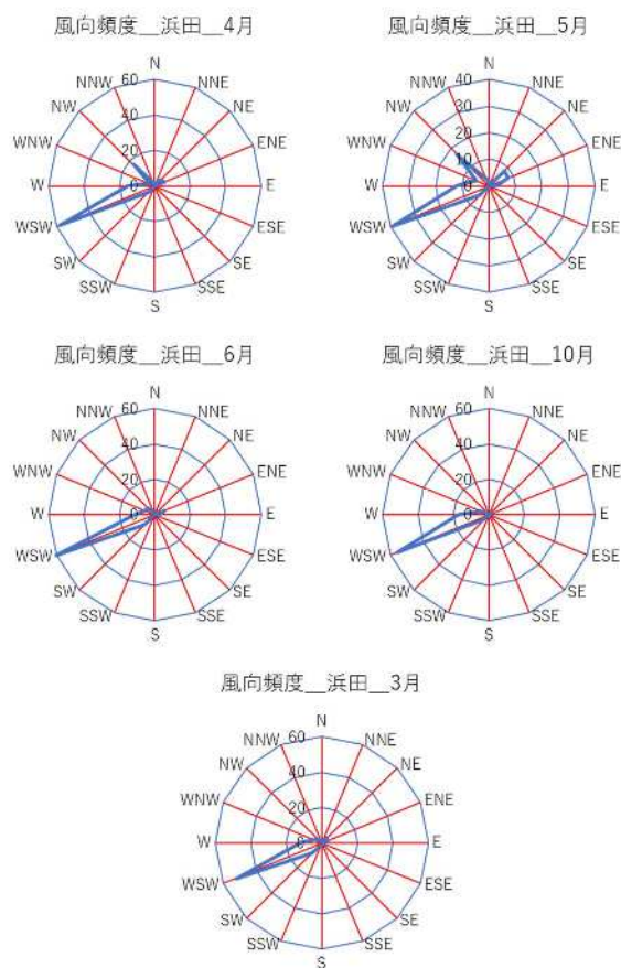
図 4 2023 年度の浜田の光化学 0x 濃度 0.06ppm 以上観測時における風向頻度
