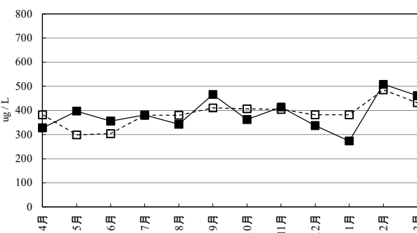
図3-3 中海の全窒素(T-N)の月別変化
