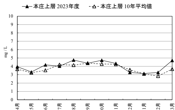
図 4-1 本庄のCODの月別変化
