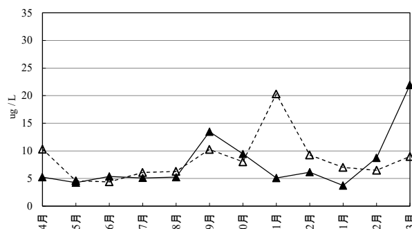
図 4-2 本庄のクロロフィルa(Chl-a)の月別変化
