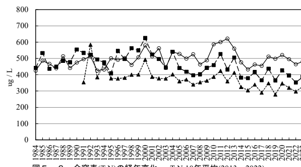
図 5-3 全窒素(T-N)の経年変化
