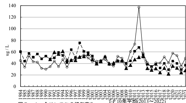
図 5-4 全リン(T-P)の経年変化
