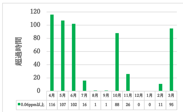
図 2 2023年度の浜田において光化学 O_x の1時間値が 0.06\text{ppm} を超過した時間数
